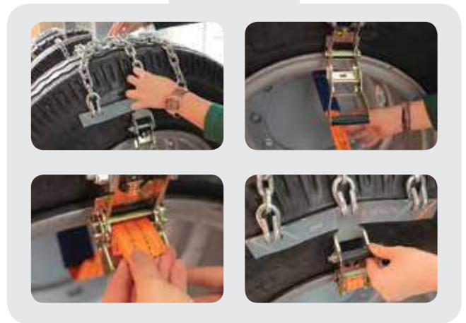
montaj / montage
