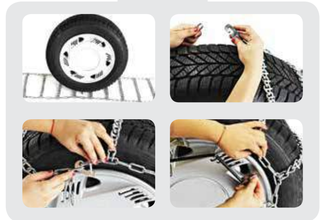
montaj / montage
